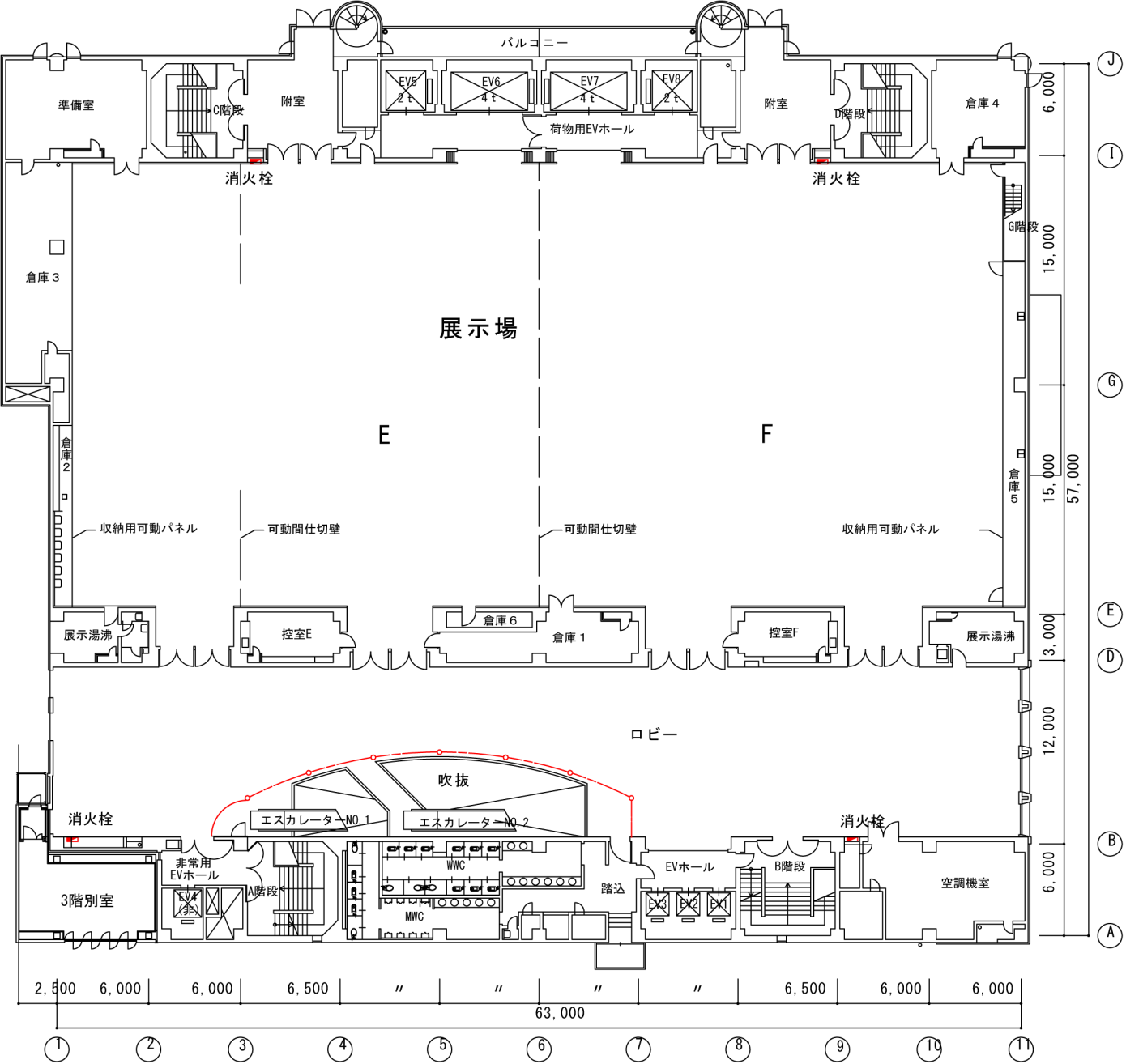
3階平面図 1/400
